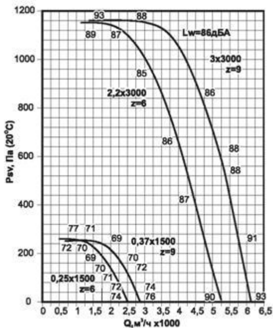
Аэродинамическая характеристика ВКРФ 3,55
