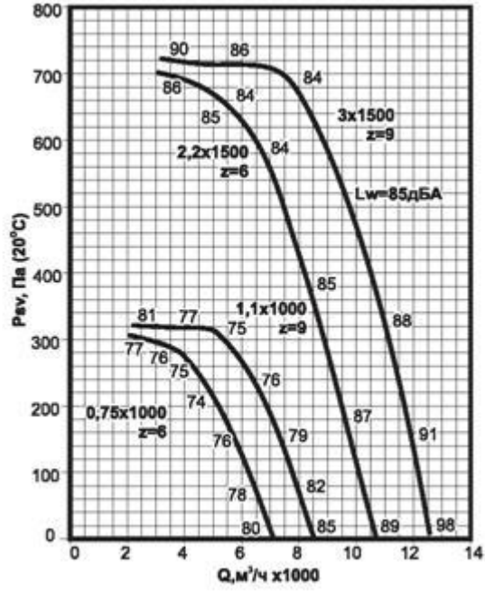
Аэродинамическая характеристика ВКРФ 6,3
