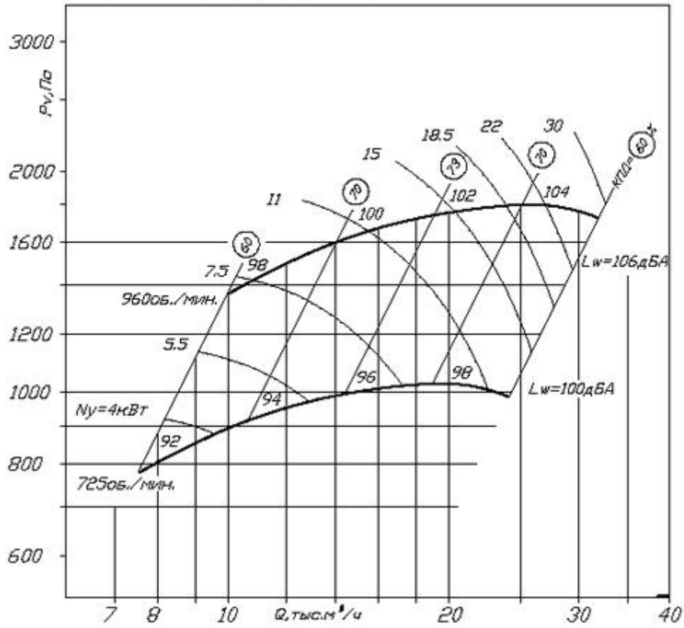
ВЦ 14-46-6.3 схема 1
