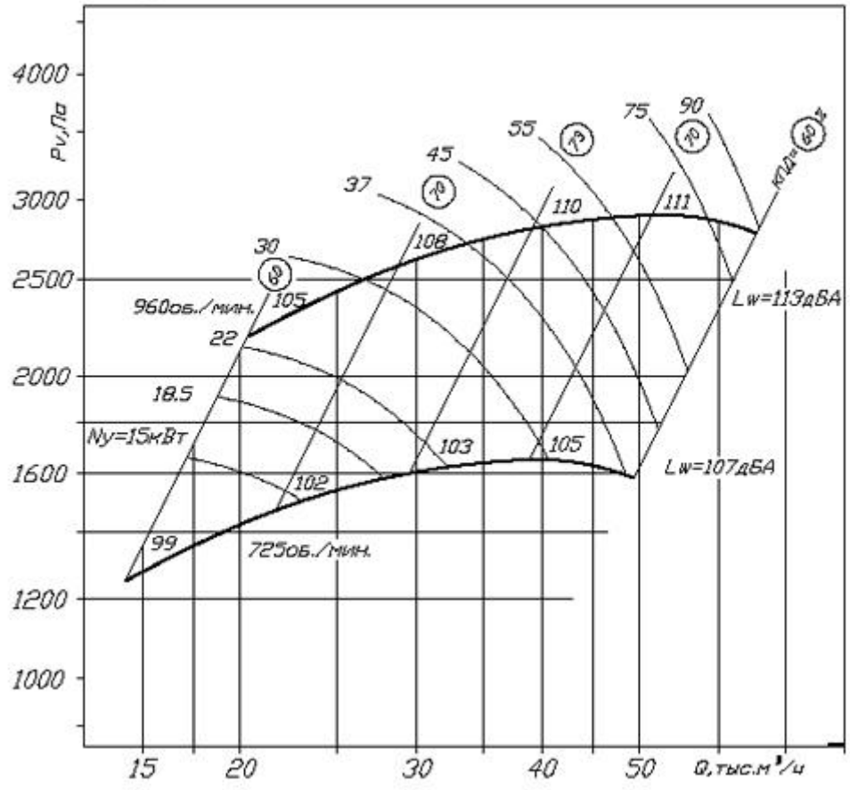
ВЦ 14-46-8 схема 1
