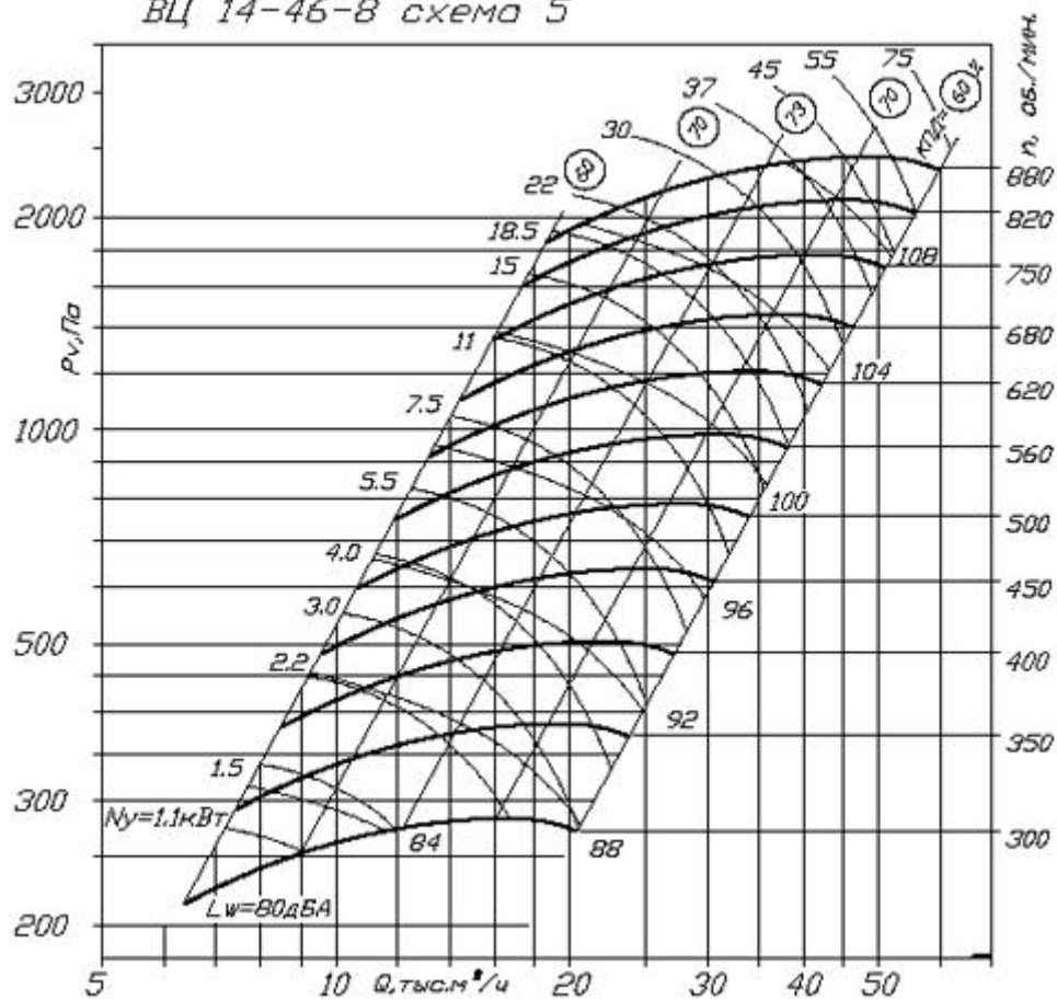
ВЦ 14-46-8 схема 5
