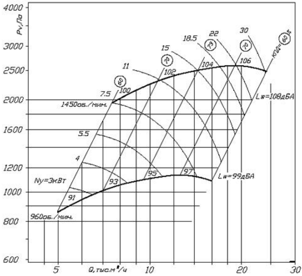
ВЦ 14-46-5 схема 1
