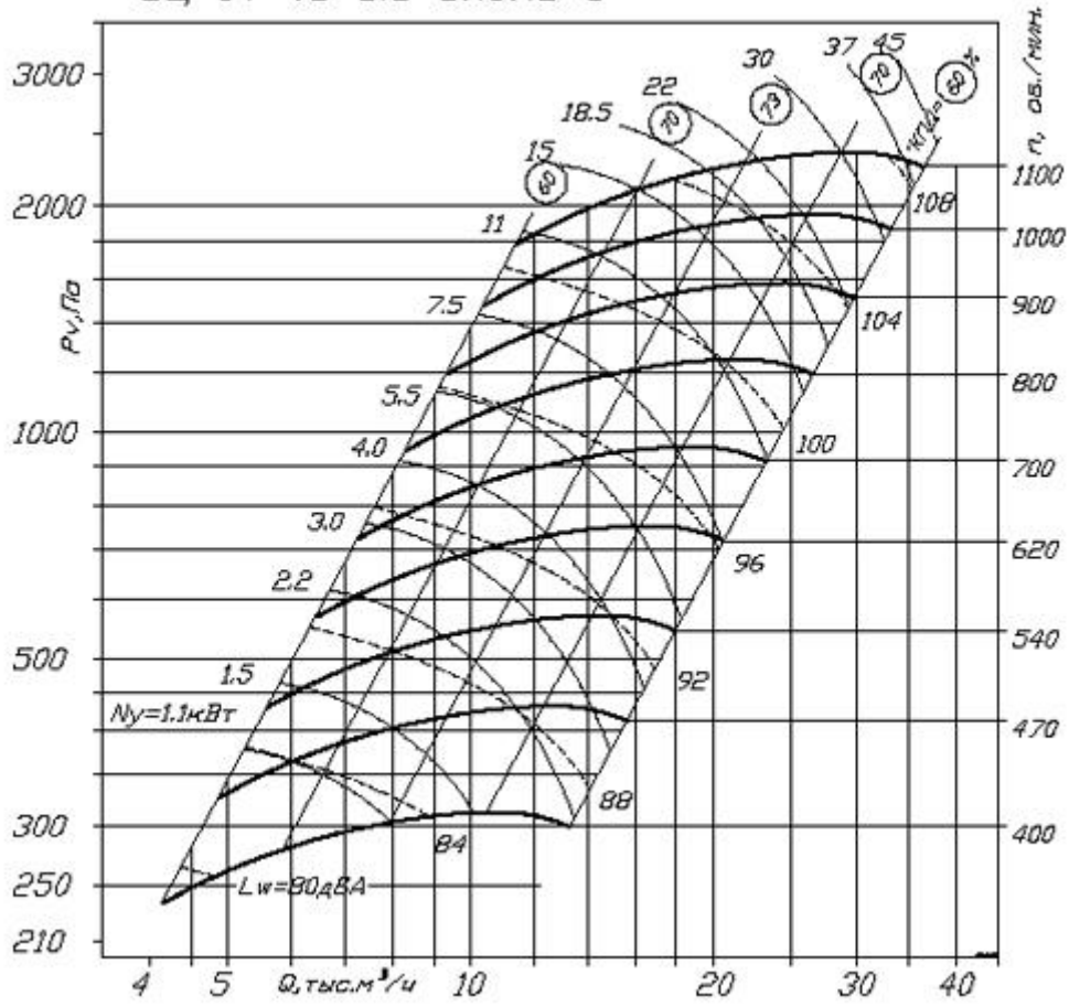
ВЦ 14-46-6.3 схема 5
