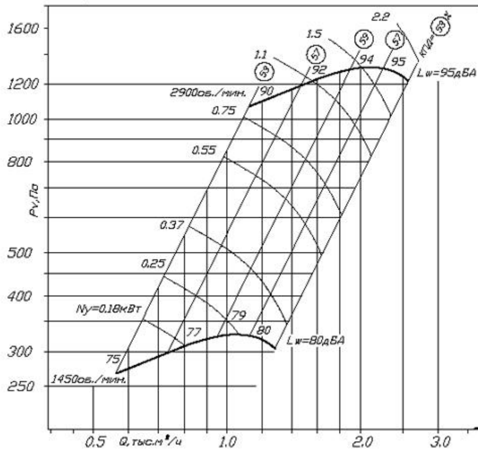
ВЦ 14-46-2 схема 1
