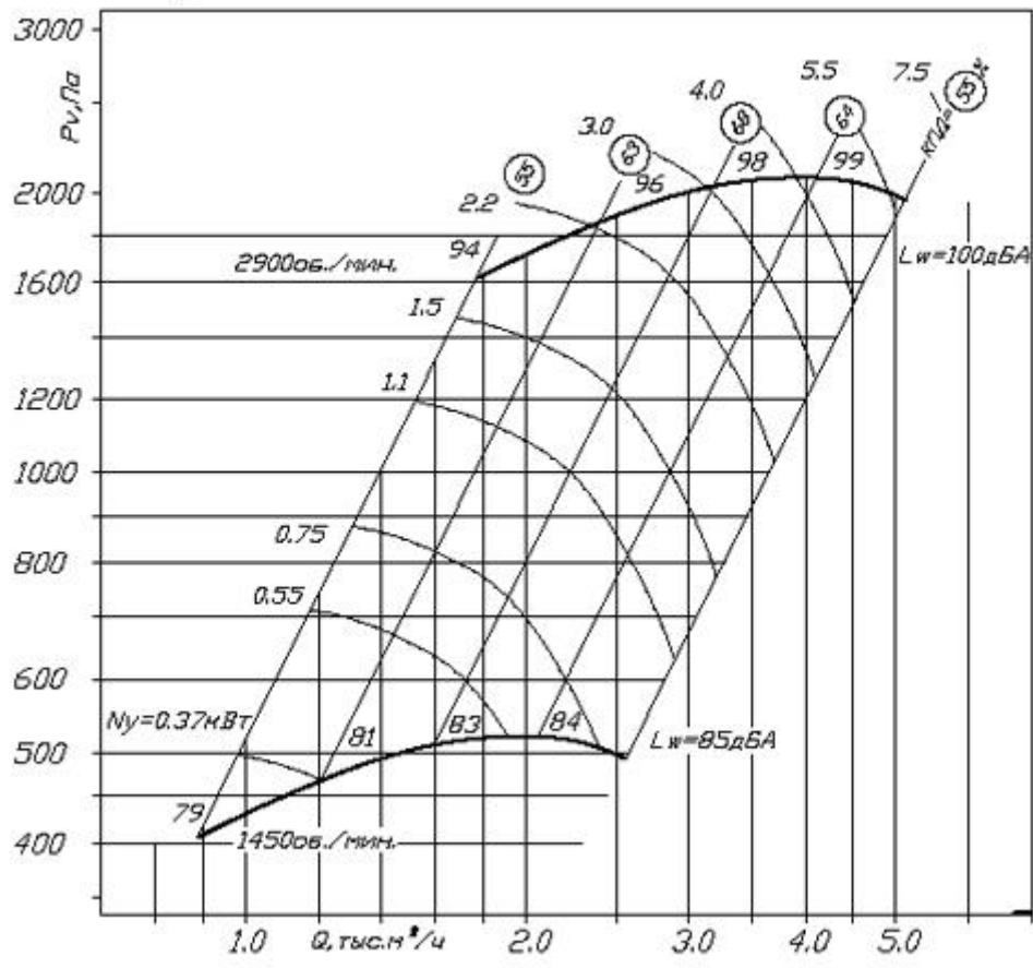
ВЦ 14-46-2.5 схема 1
