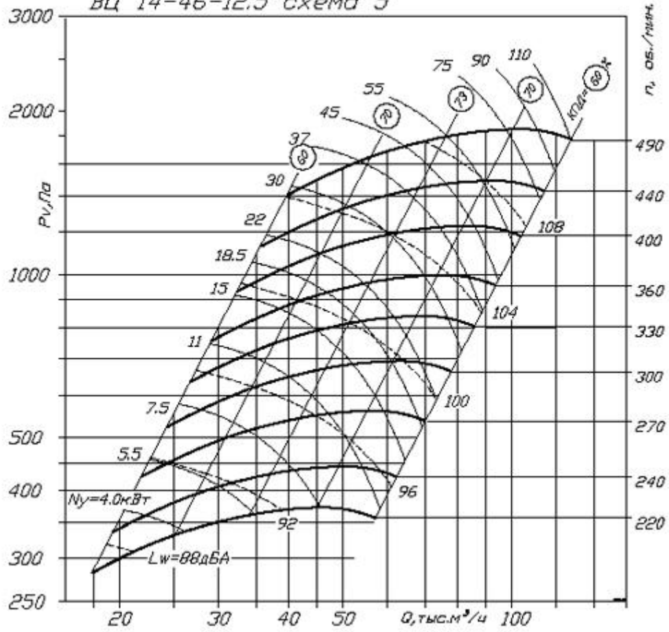
ВЦ 14-46-12.5 схема 5
