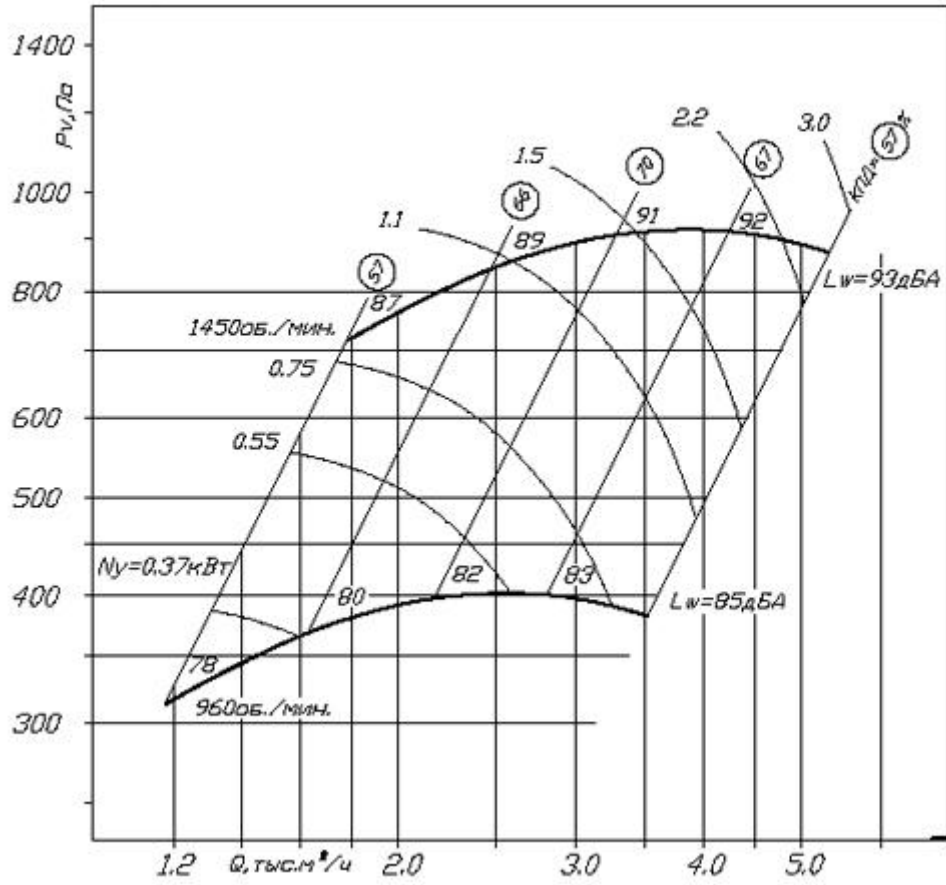
ВЦ 14-46-3.15 схема 1
