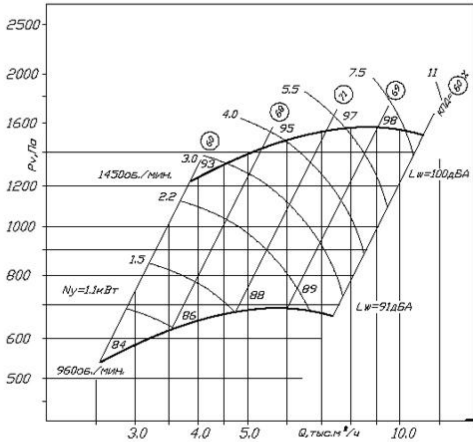
ВЦ 14-46-4 схема 1
