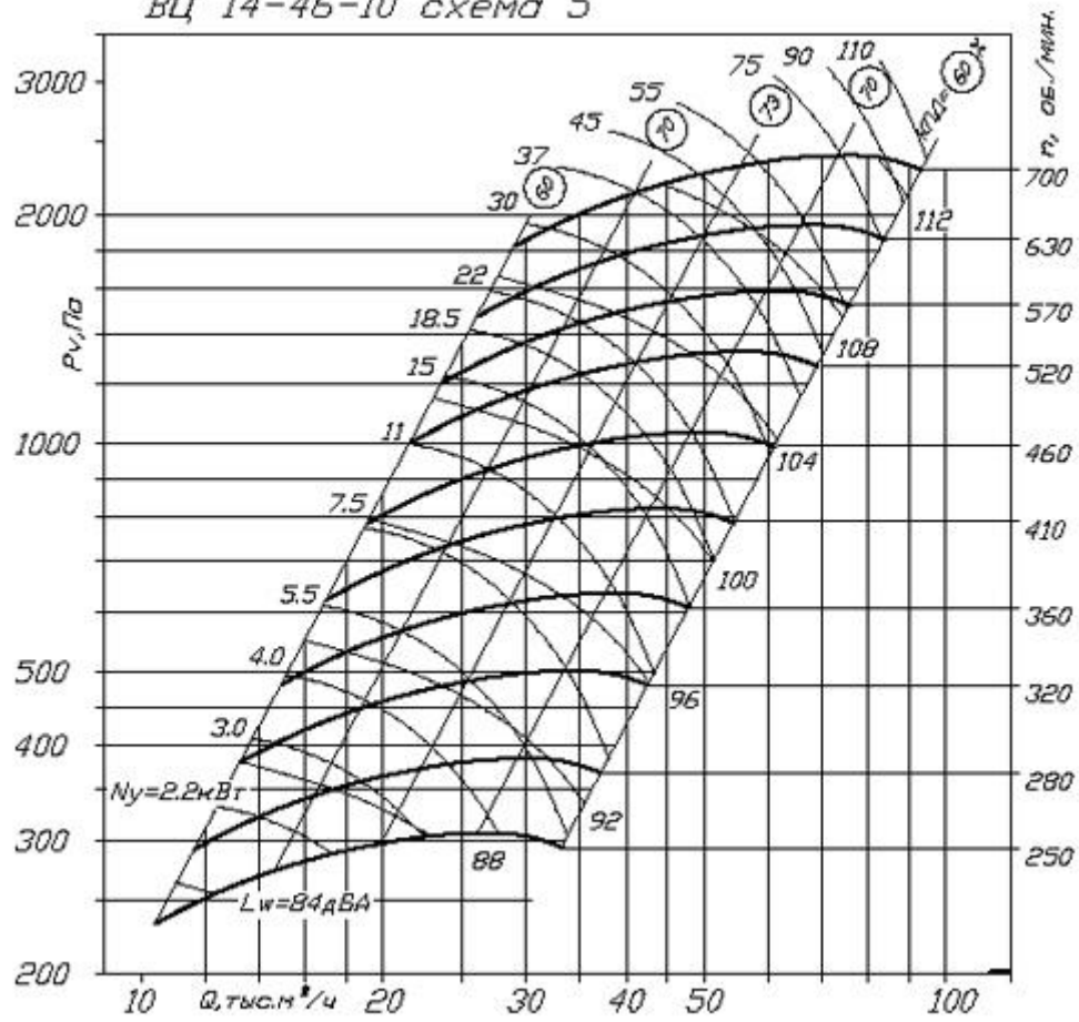
ВЦ 14-46-10 схема 5
