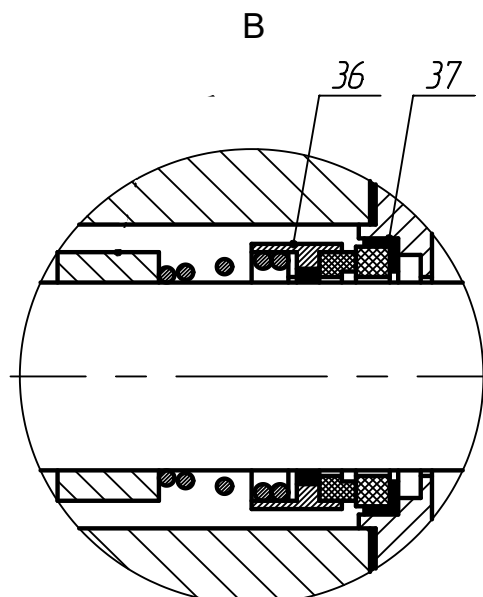
Рисунок Б.2 Уплотнение торцовое производства АО «ГМС Ливгидромаш»
