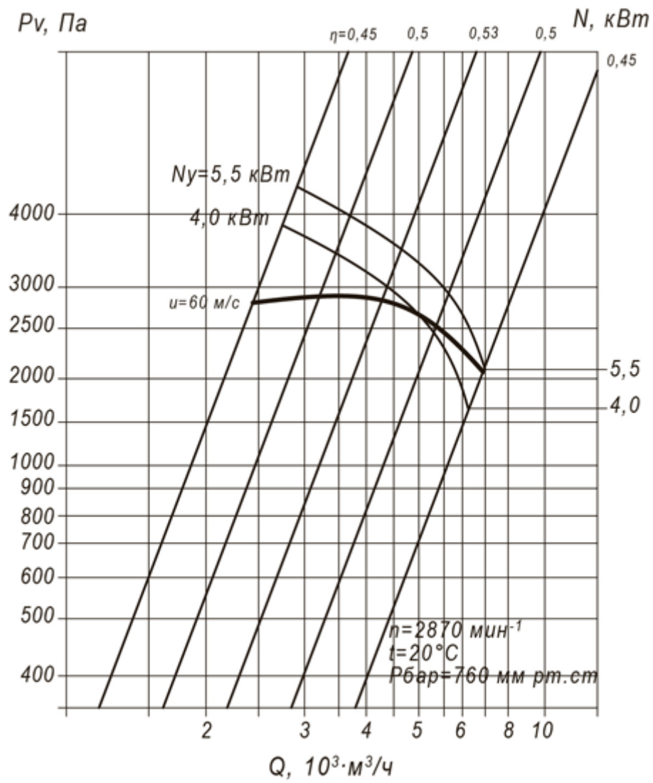
Аэродинамическая характеристика ВЦП 7-40 №5
