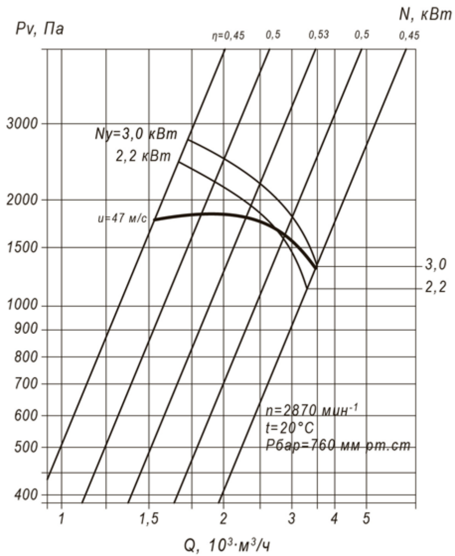
Аэродинамическая характеристика ВЦП 7-40 №4
