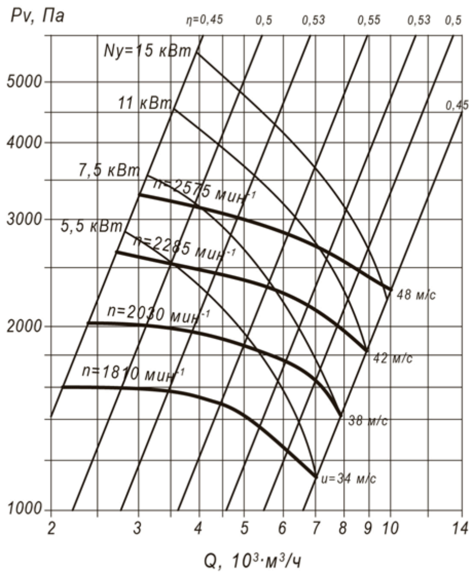
Аэродинамическая характеристика ВЦП 7-40 №6,3
