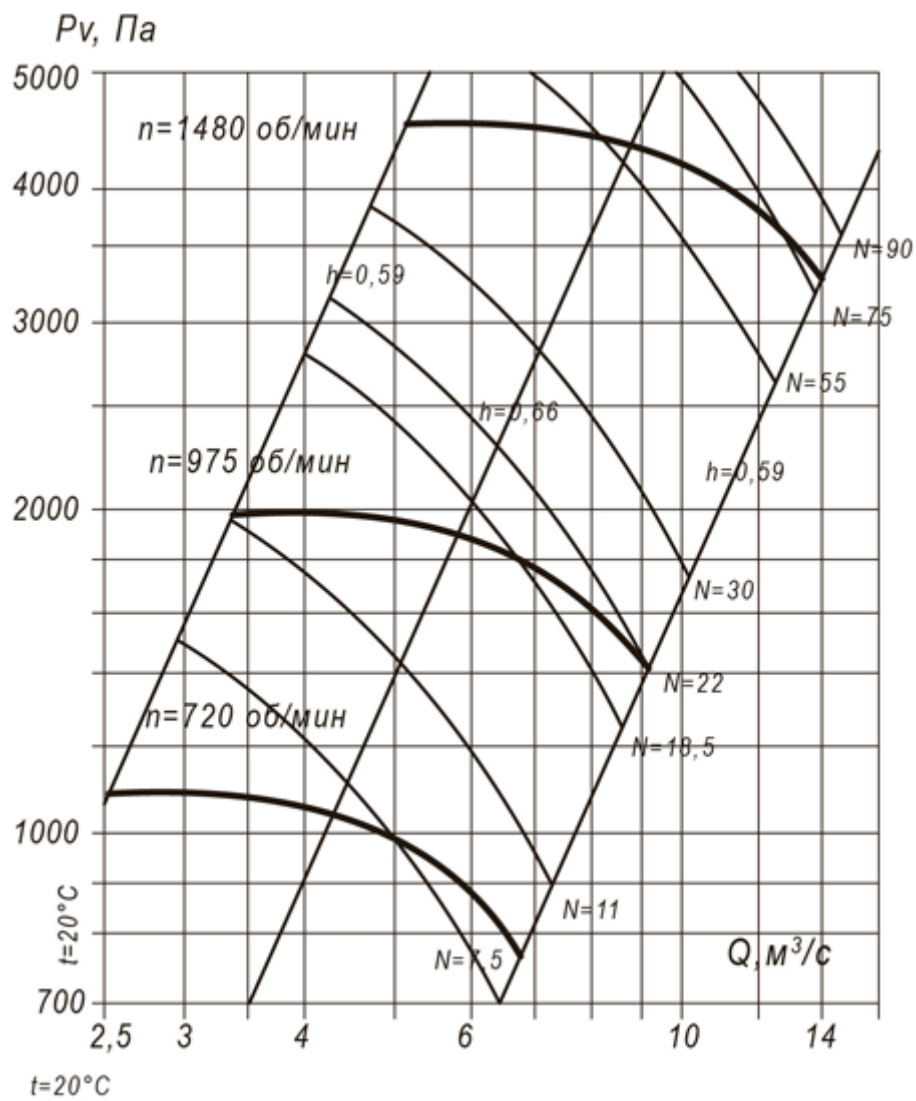
Аэродинамическая характеристика ВЦП 7-40 №12,5
