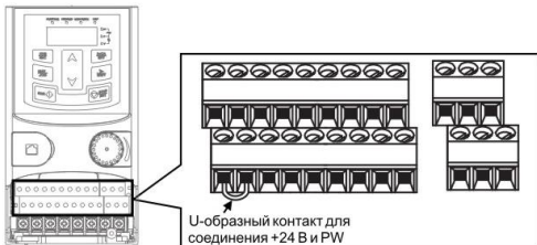
Рис. 4-10. U-образный контакт
